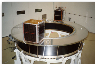
1995. El UPM-Sat 1 sobre la plataforma de cargas auxiliares del lanzador Ariane
